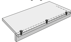
Blendenbefestigung
