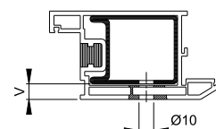
Kunststoff-Profil
