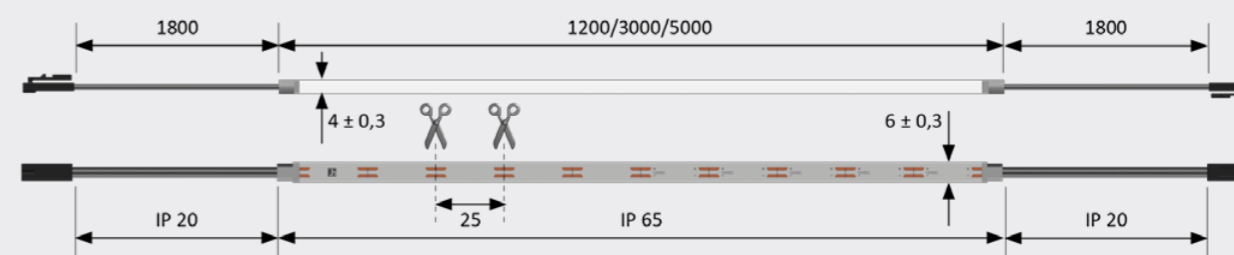
Montagezeichnung Individuell kürzbar
