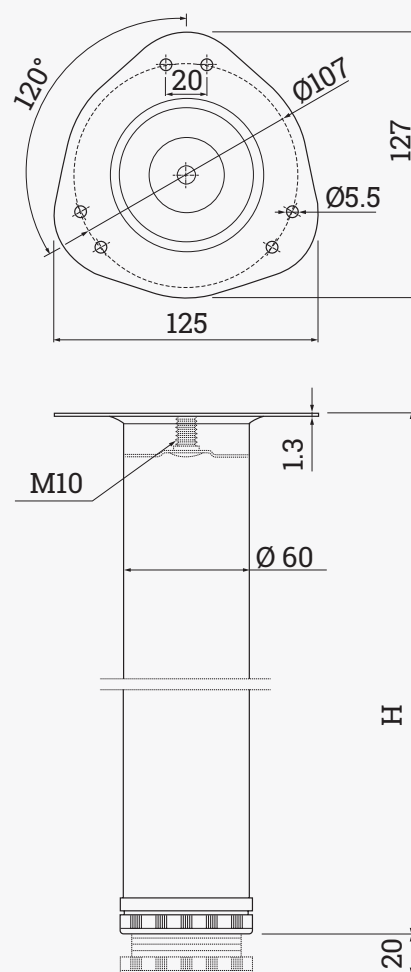
Technische Zeichnung
