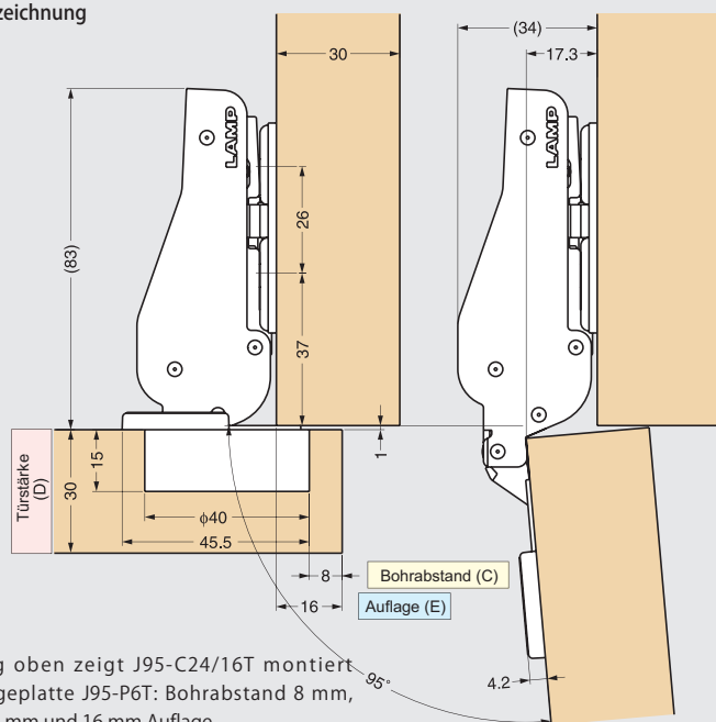
Abbildung oben zeigt Topfscharnier und Montageplatte
