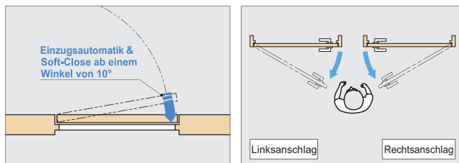
Rechtsseitige Ansicht
