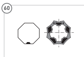
Achtkantwelle 50 mm
