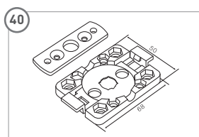
Schnellmontagelager-PVC*
